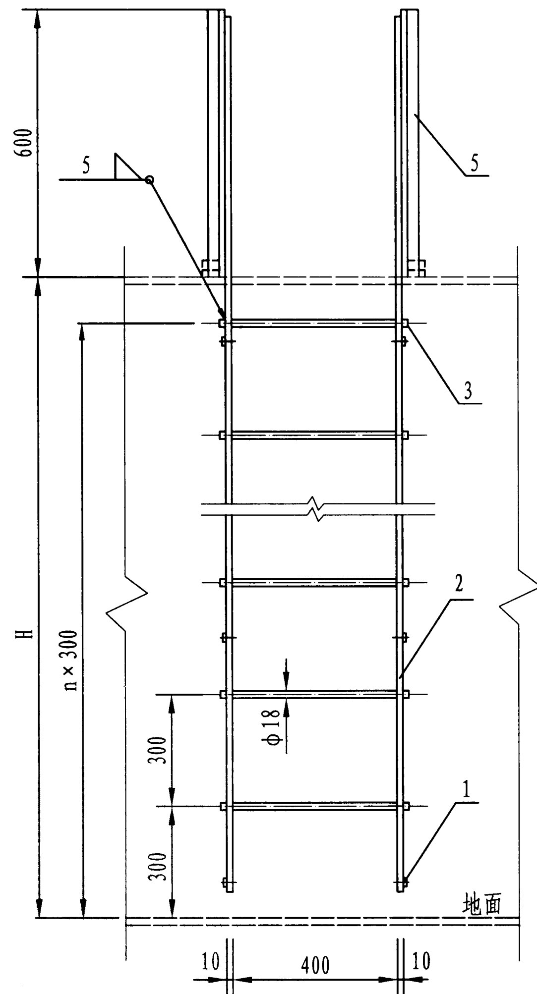
立面图
