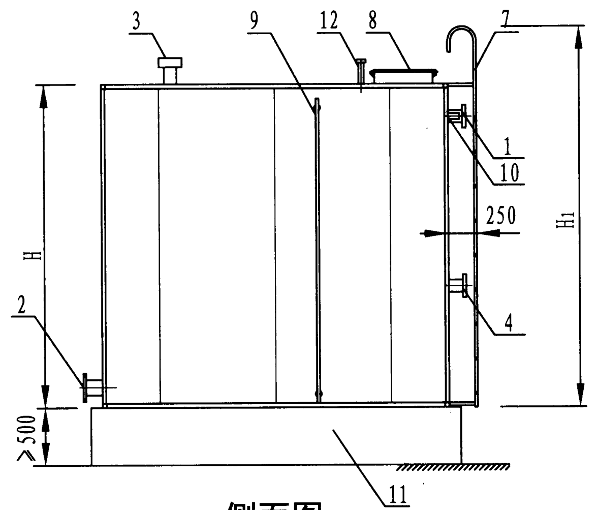
侧面图
