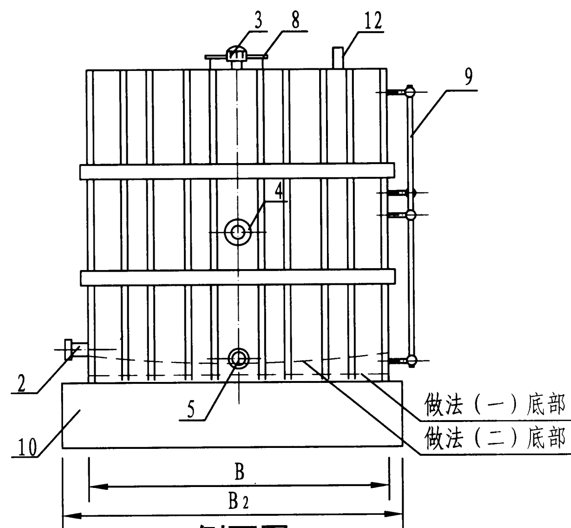
侧面图
