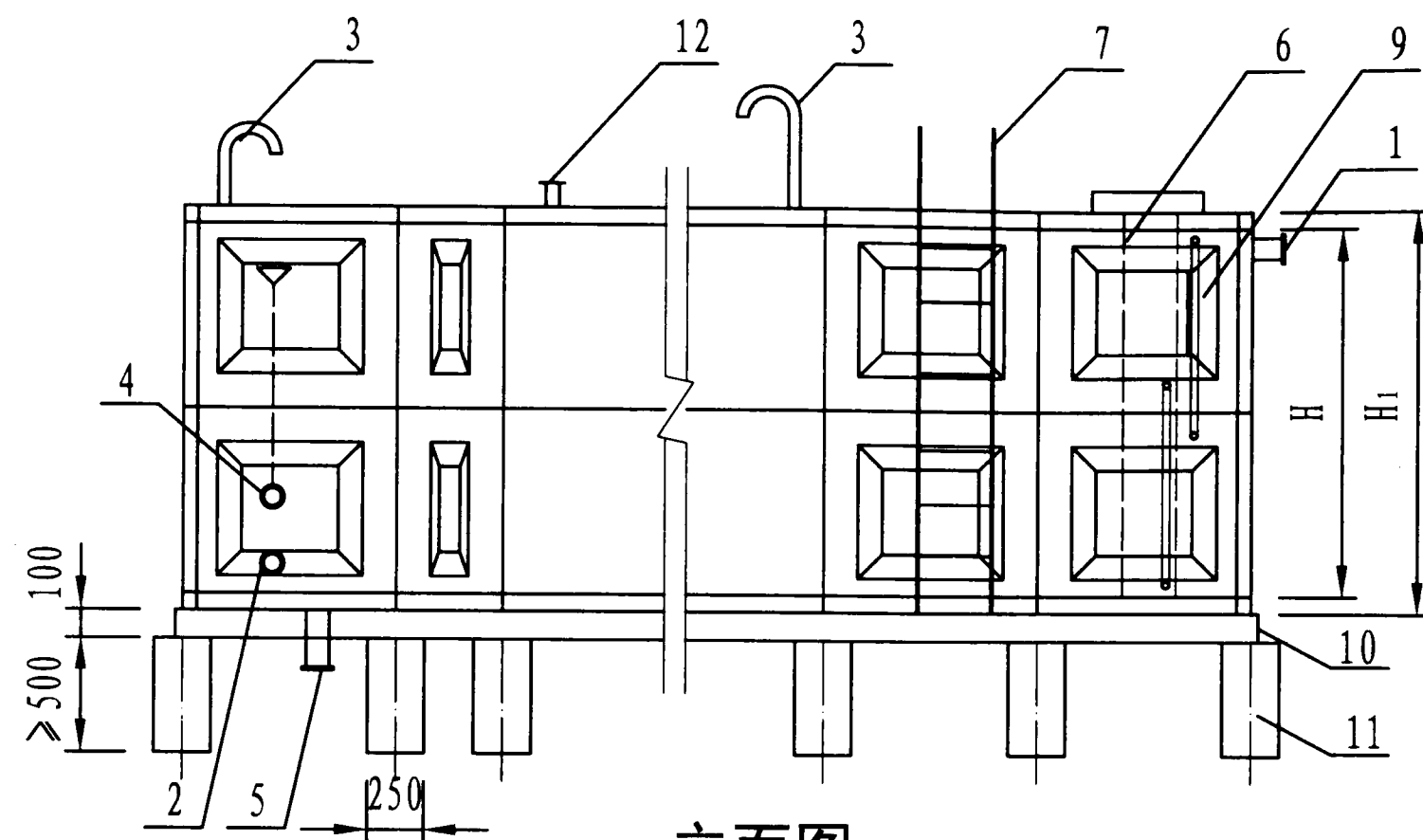
立面图
