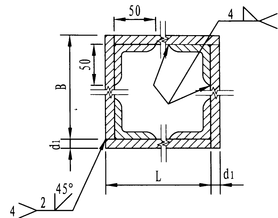
箱壁拼板图
