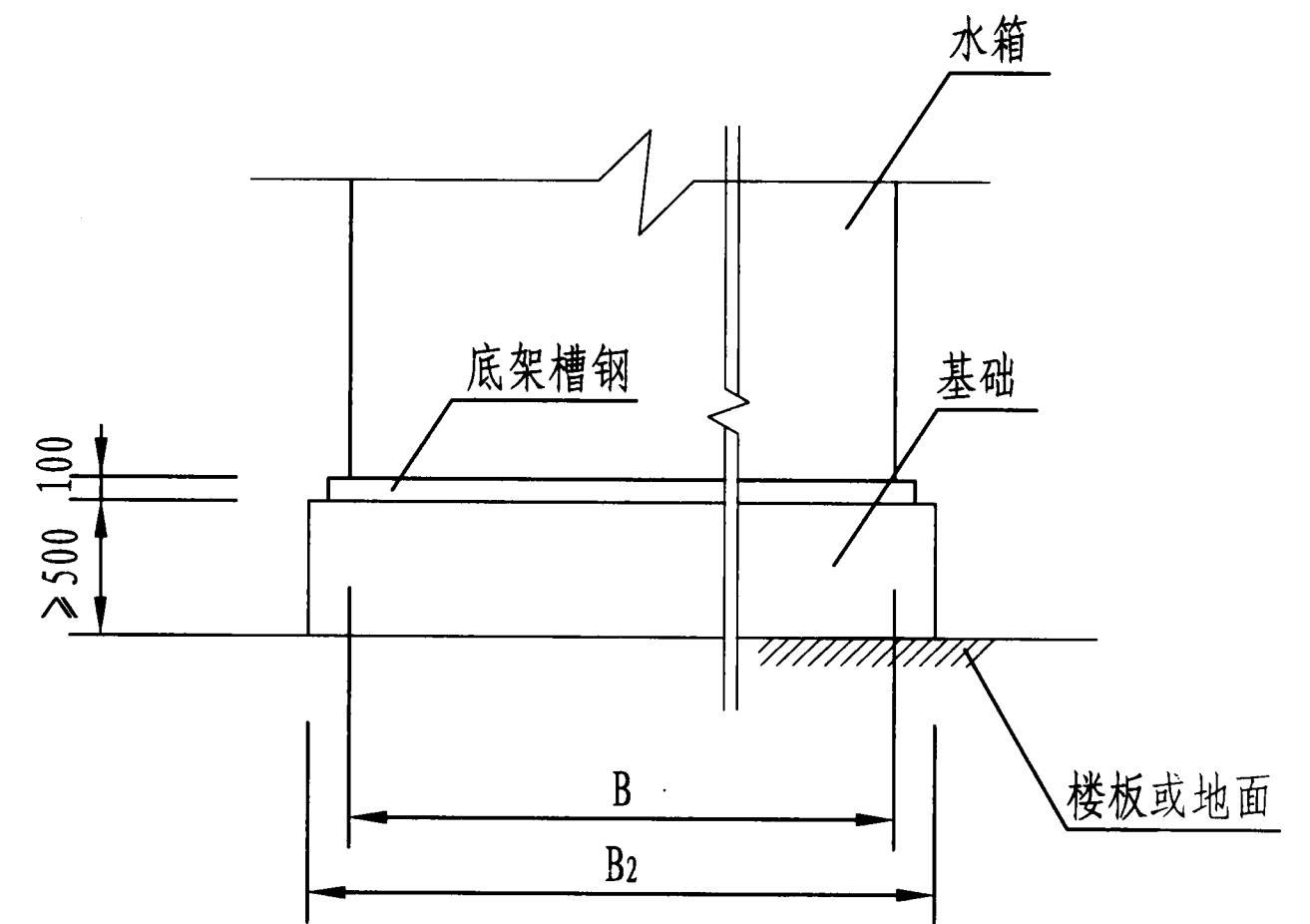
侧立面
