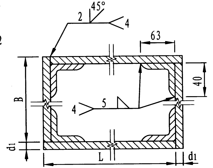
箱壁拼板图
