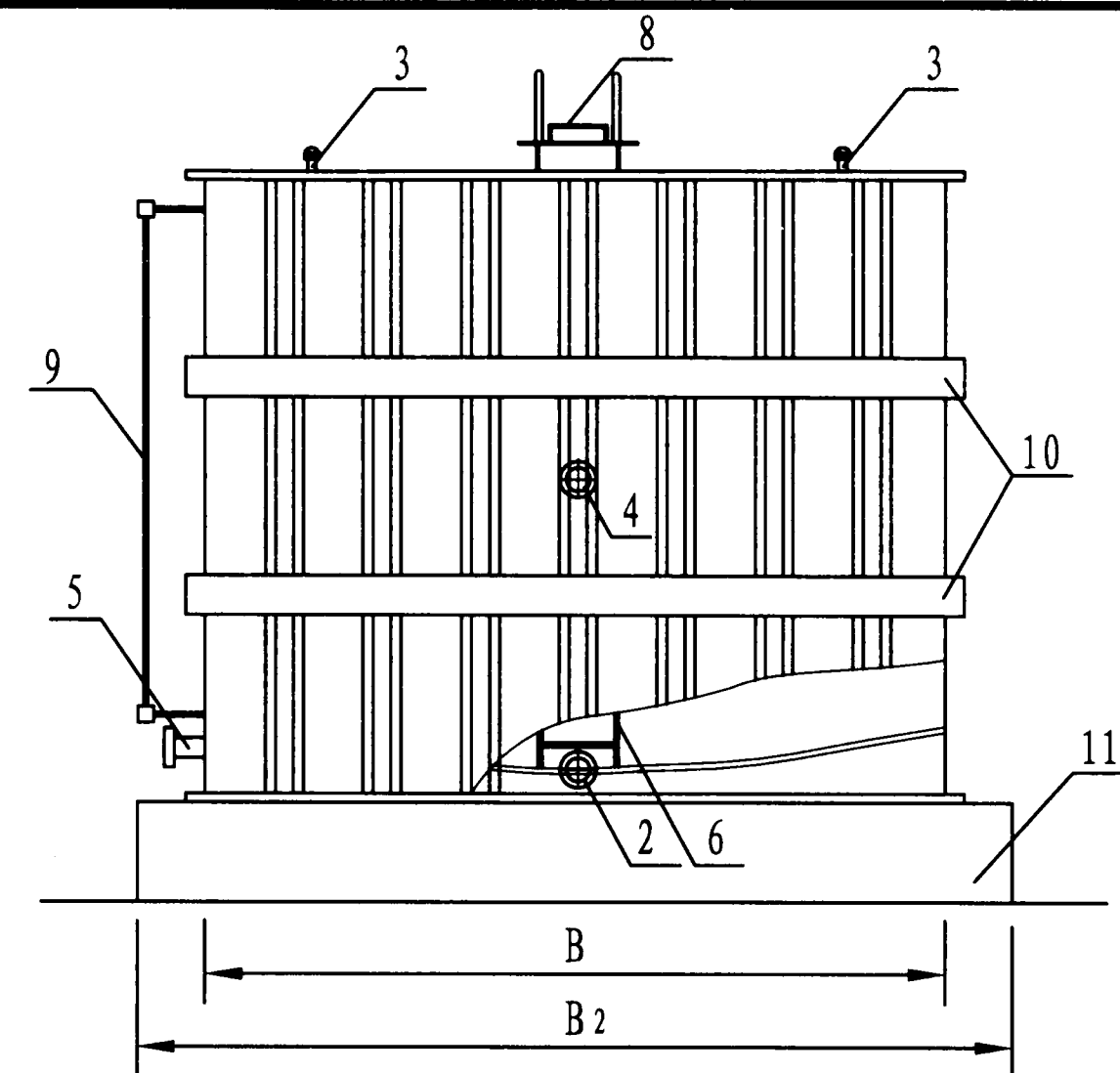
侧立面
