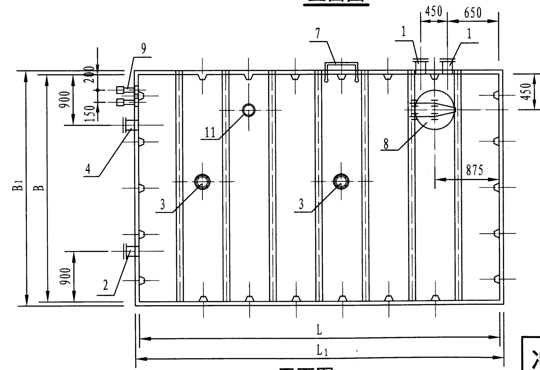
平面图
