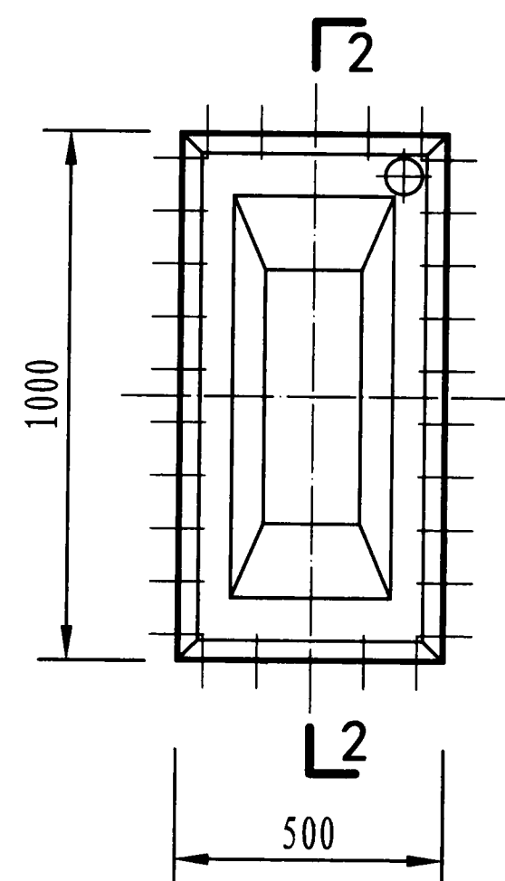
1000×500单板平面图
