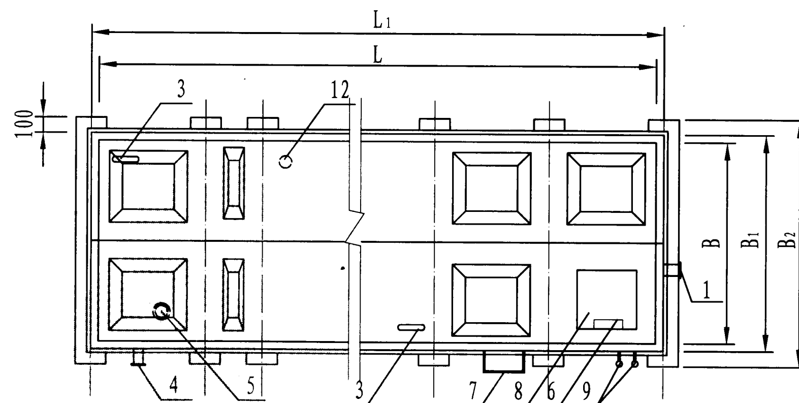
平面图
