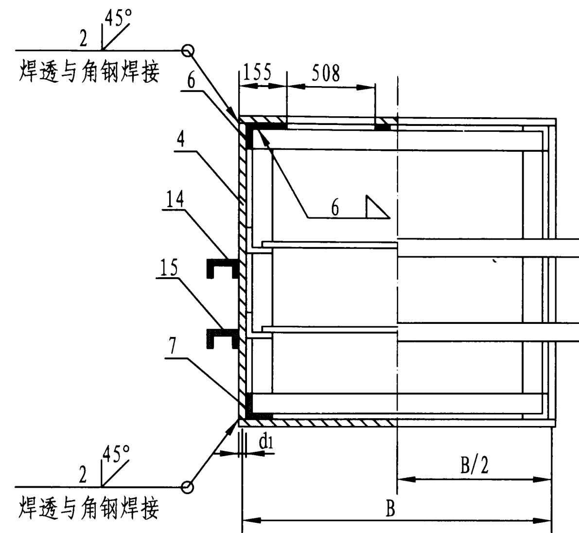
2-2剖面图
