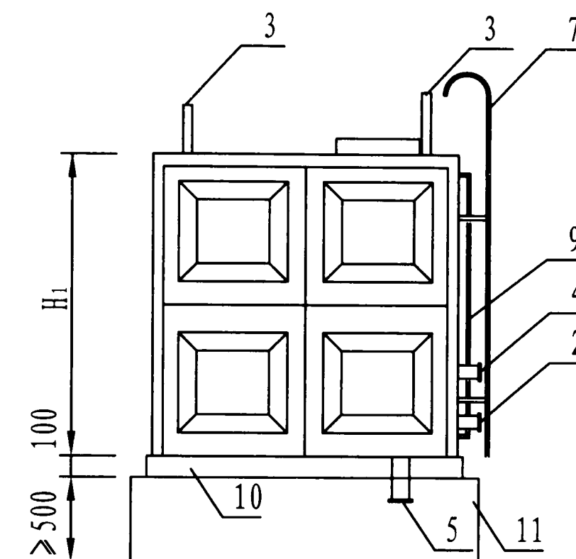
侧面图
