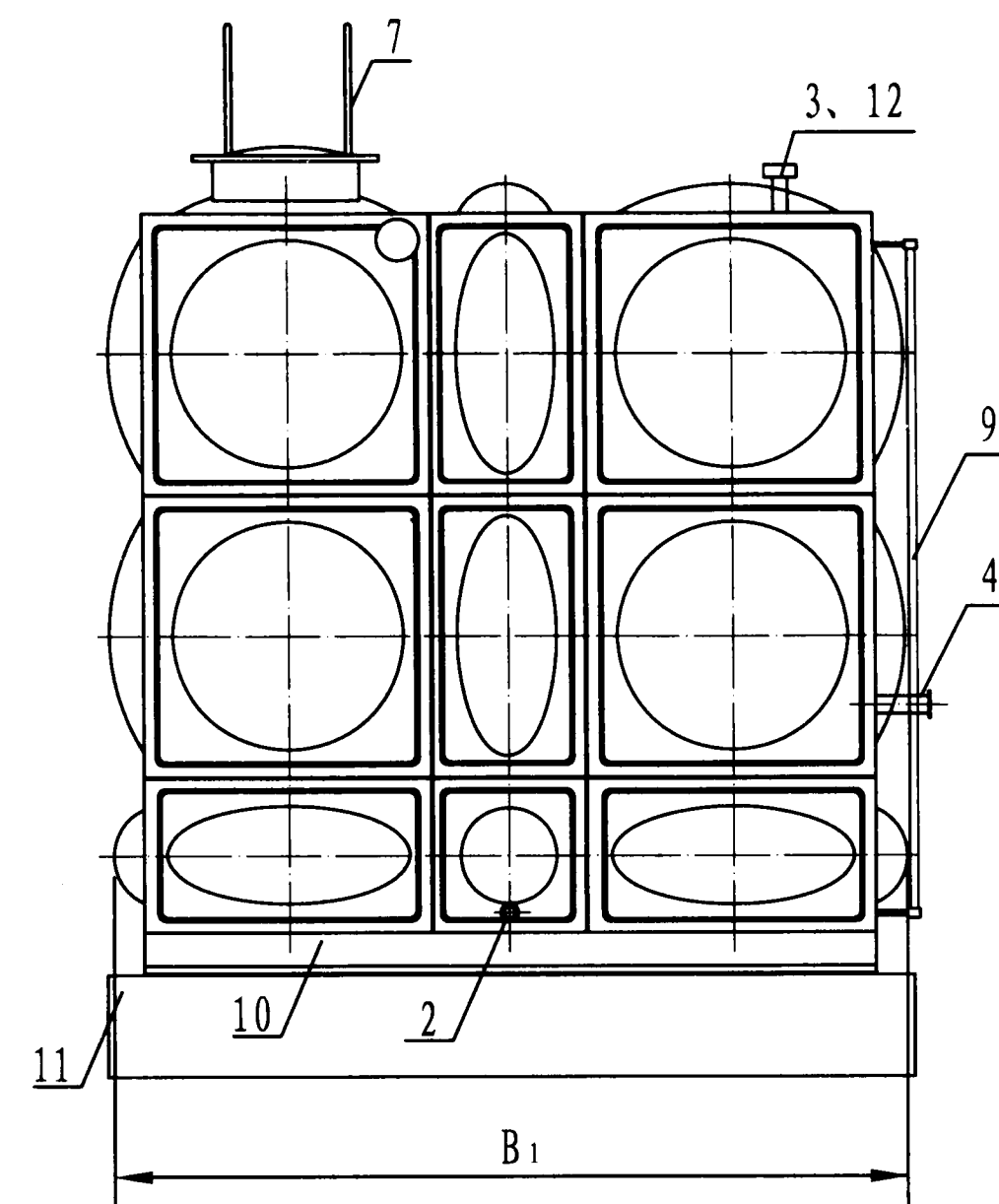
侧立面
