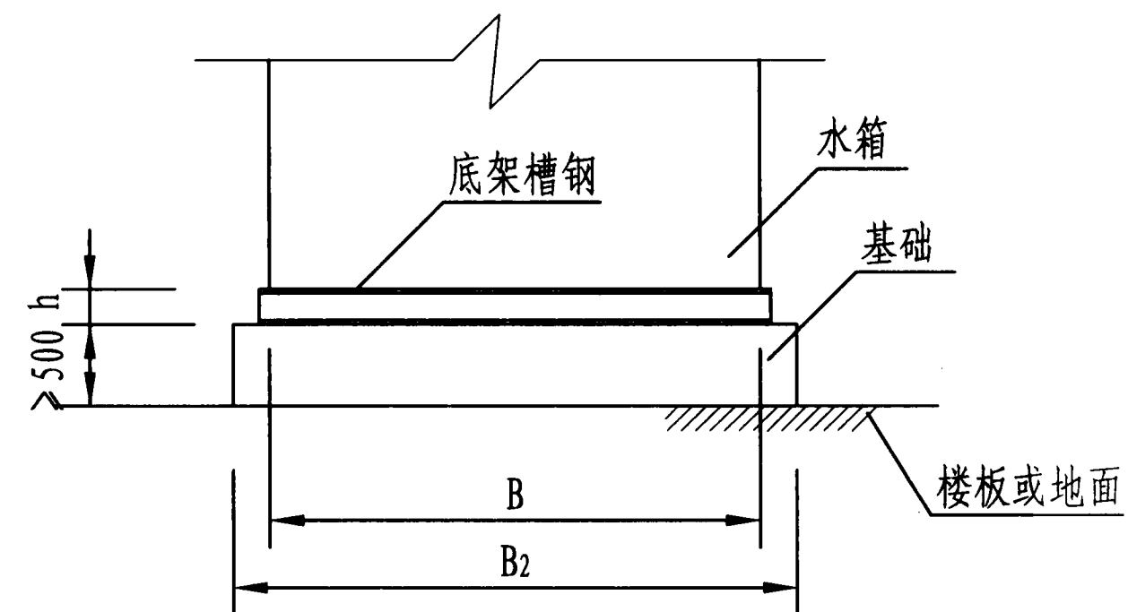
侧立面
